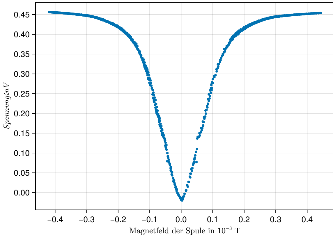
Eichkurve von Sensor 2
